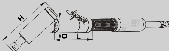
GDB 070-...BX-Winkel 120°
