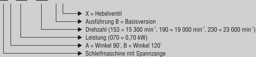
GDA 070-...BX-Winkel 90°
