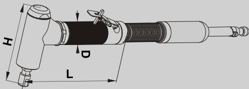
GDA 070-...BX-Winkel 90°
